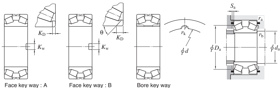
Face key way : A
